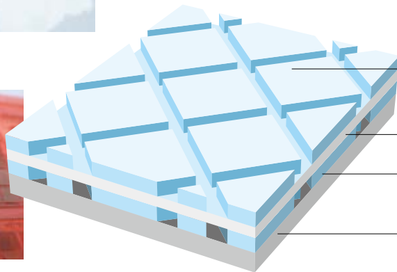
3M™ クッションマウント™ プラス 版固定用テープ Eシリーズ 構造図
